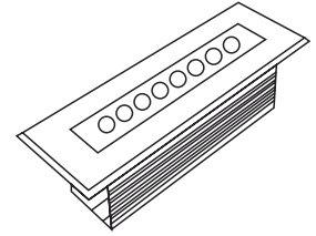
* Delik Ebat: 28x5x6,5 cm * Çerçeve Ebat: 34x9 cm
