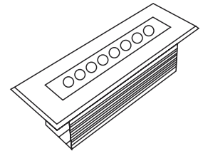
* Delik Ebat: 99x5x6,5 cm * Çerçeve Ebat: 103x9 cm
